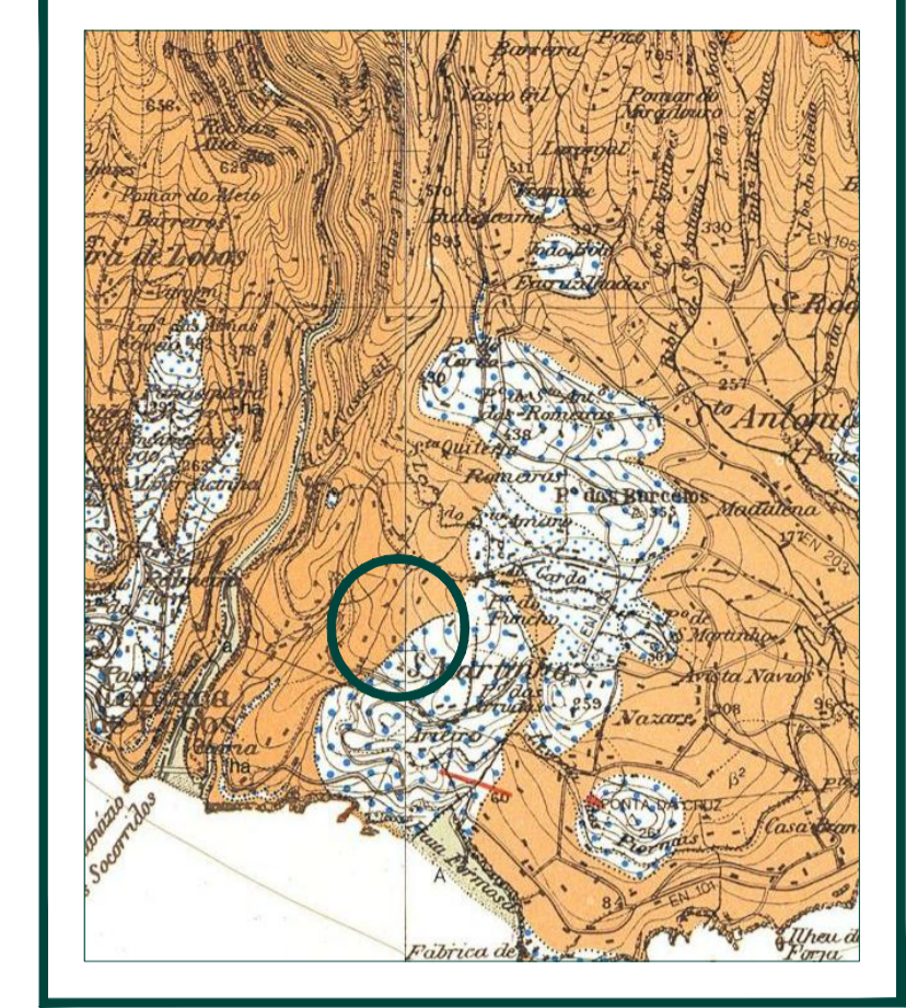
EXTRACTO DA CARTA GEOLÓGICA DE PORTUGAL Folha A e Folha B (Escala original: 1/50 000)
