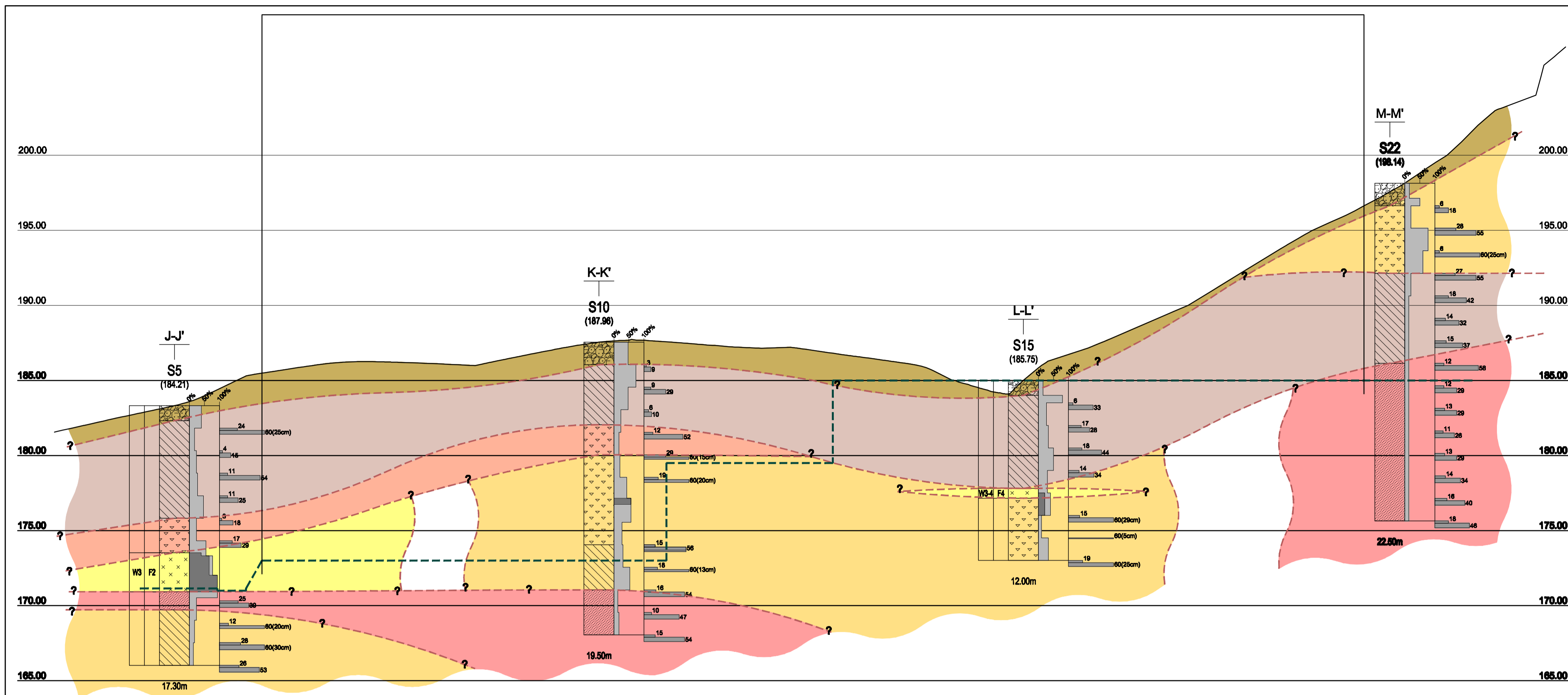
PERFIL INTERPRETATIVO D-D' PLANIFICADO Escala: V: 1/200 H: 1/500
