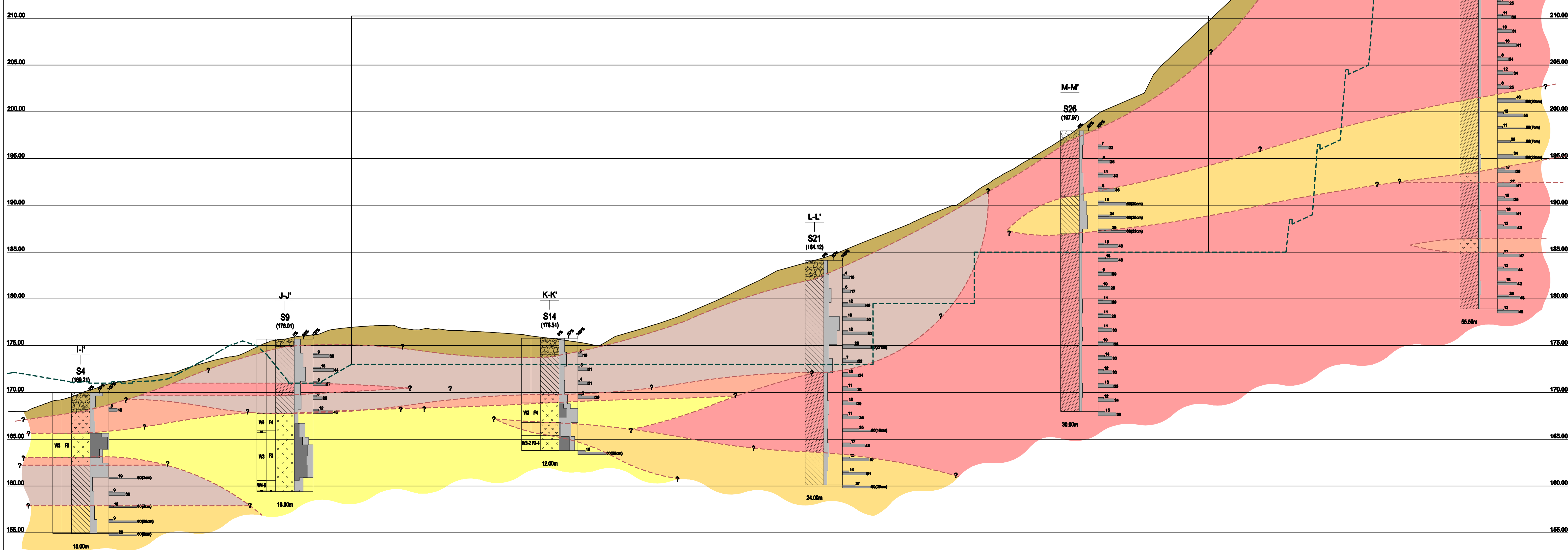
PERFIL INTERPRETATIVO E-E' PLANIFICADO Escala: V: 1/200 H: 1/500
