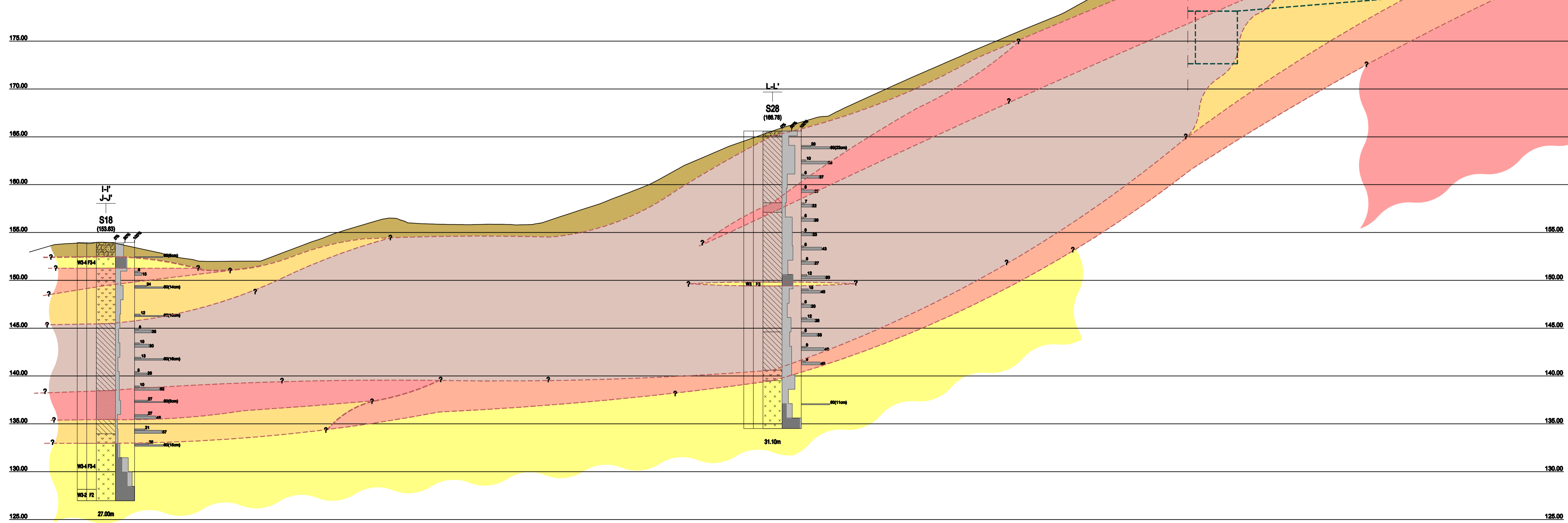
PERFIL INTERPRETATIVO H-H' PLANIFICADO Escala: V: 1/200 H: 1/500
