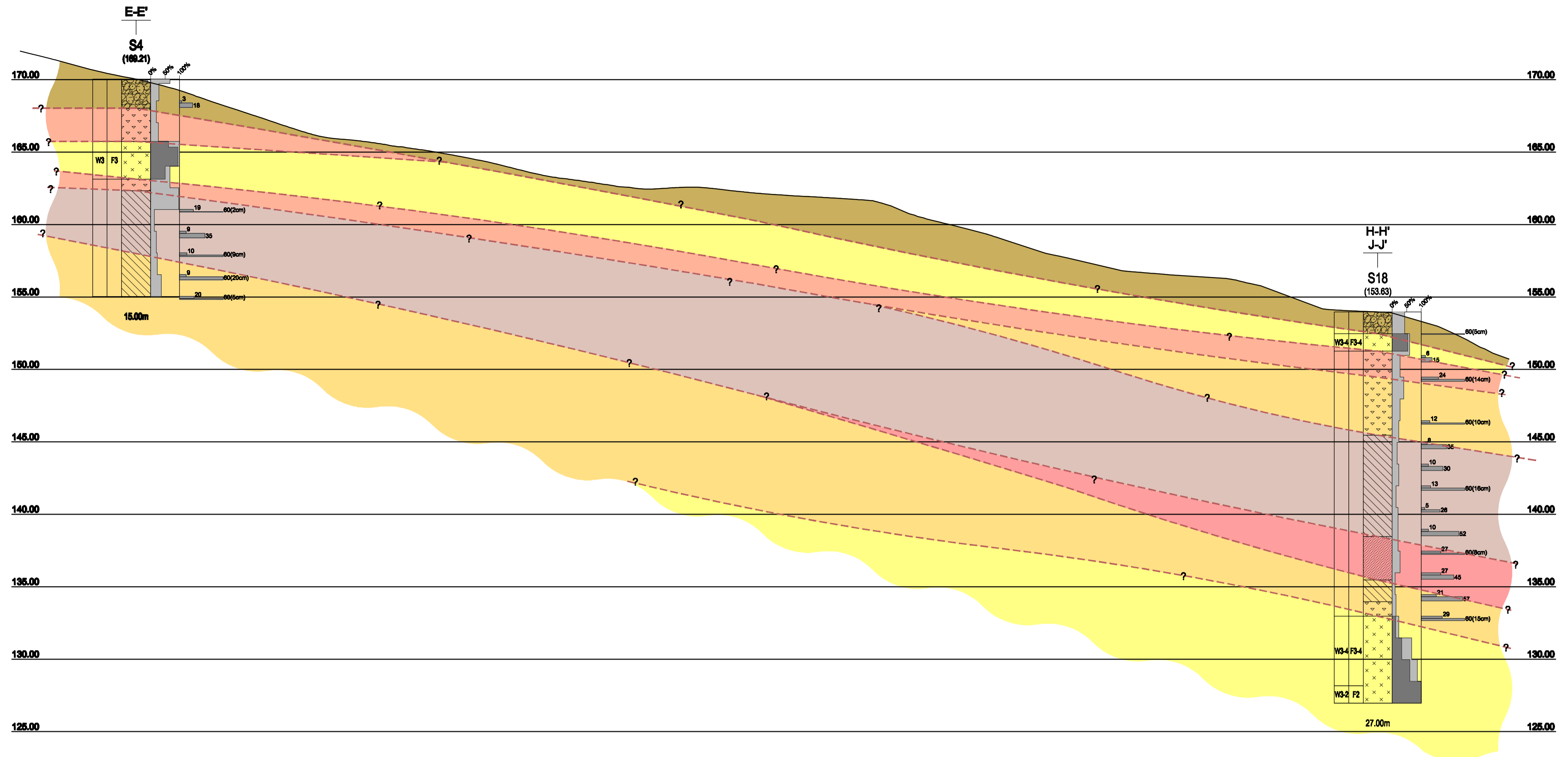
PERFIL INTERPRETATIVO I-I' Escala: V: 1/200 H: 1/500
