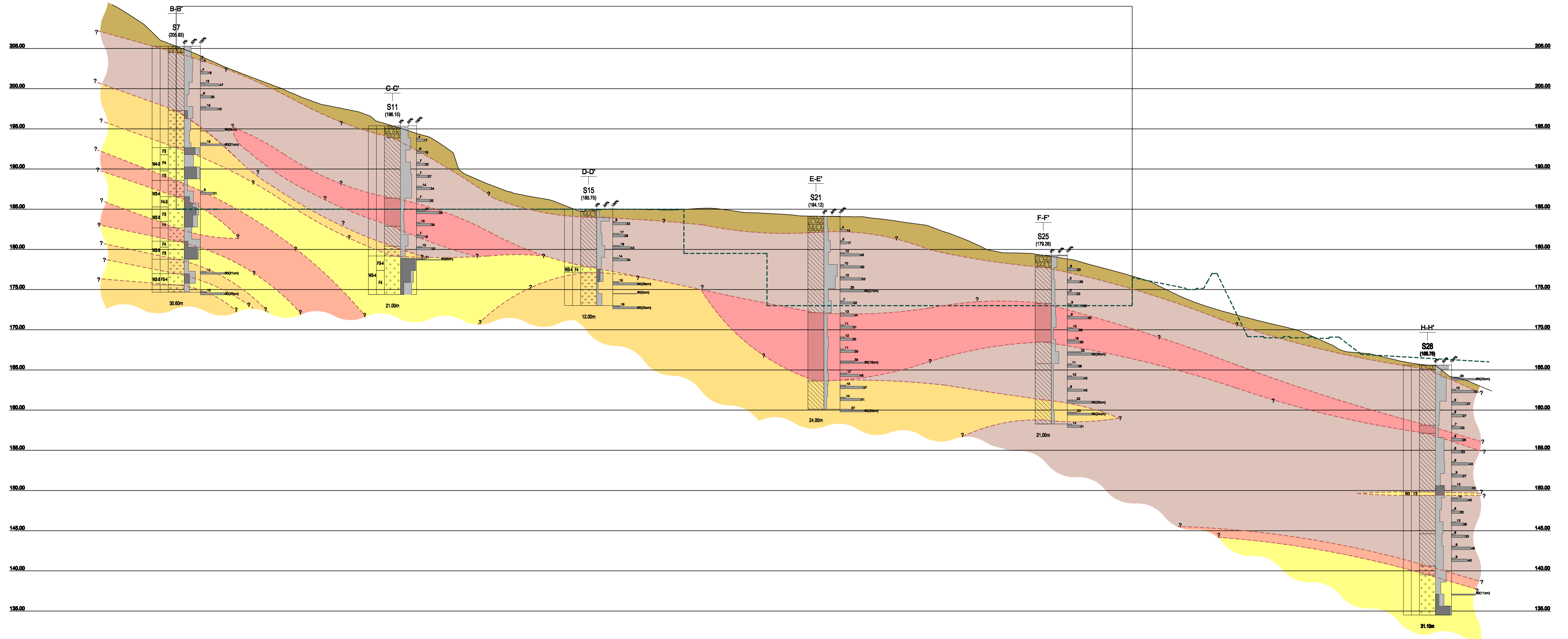
PERFIL INTERPRETATIVO L-L' PLANIFICADO Escalas : V: 1/200 H: 1/500
