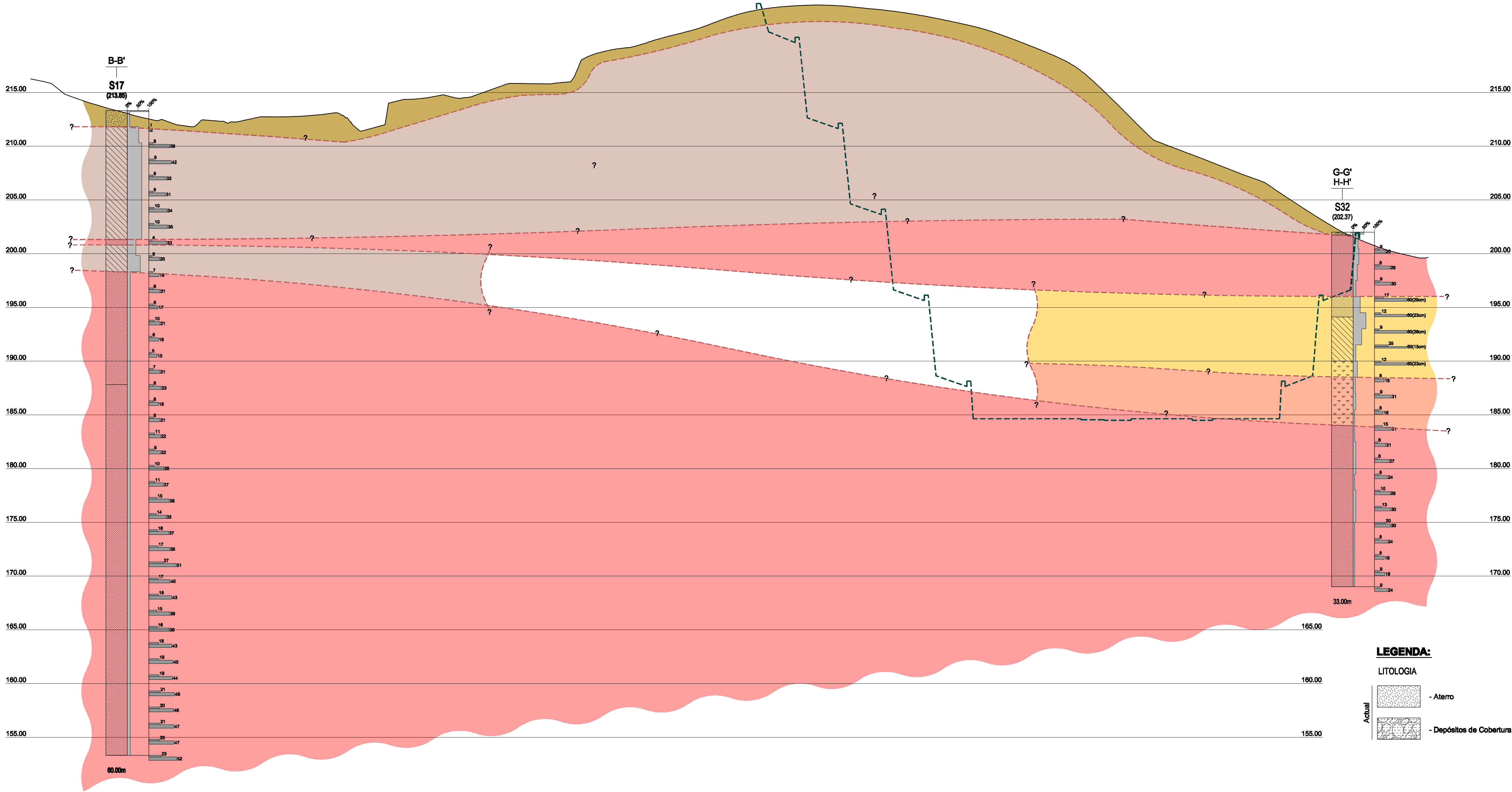
PERFIL INTERPRETATIVO O-O'
